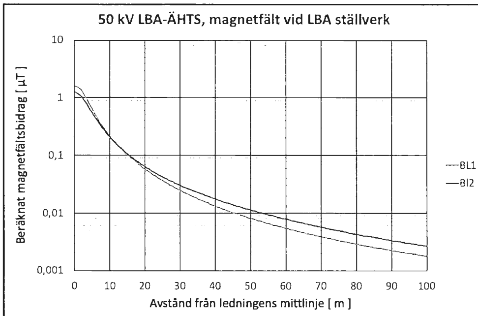
Diagram över mikroteslanivån för ställverket i relation till avstånd.
